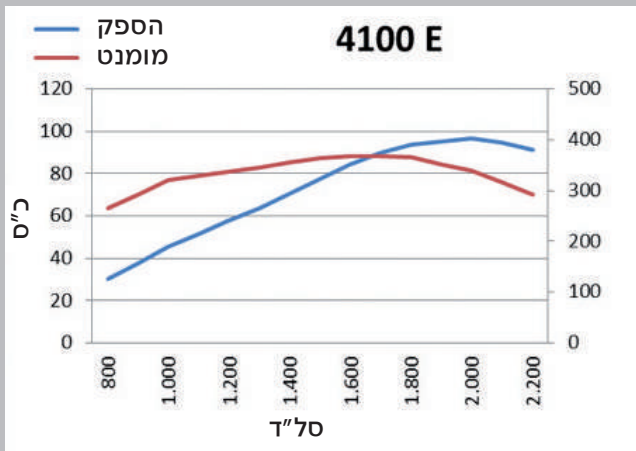
הספק מקסימלי ומומנט קבוע אפילו בתחום המהירויות הנמוכות של המנוע.
