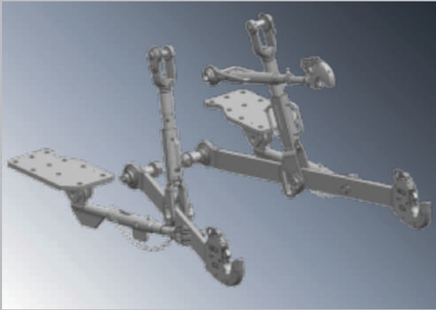
רתם אחורי עם מחברים מהירים מקטגוריה II וכושר הרמה של 3,500 ק"ג.
