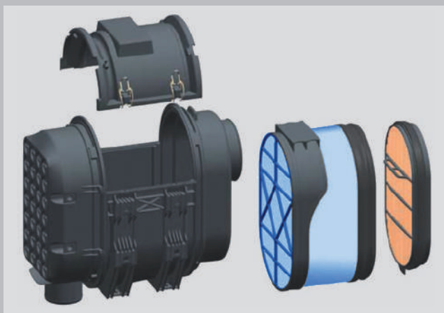
חדש: מסנן אוויר PowerCore דו-דרגתי בעל תחזוקה נמוכה עם פולט אבק.
