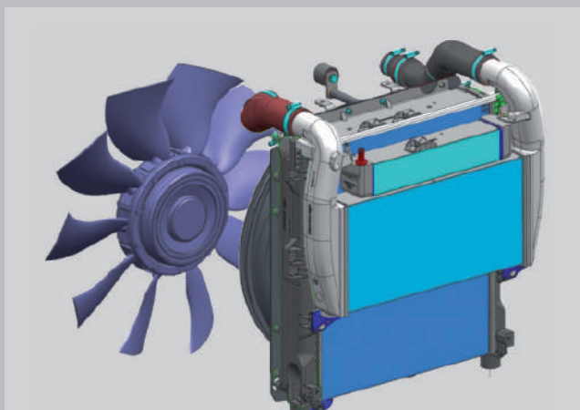
חדש: מערכת קירור עם משטח קירור מוגדל ומניפה עם מצמד צמיגות.
