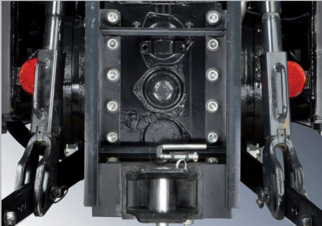
PTO: אפשר לבחור מבין 540 או 540/540ECO או 540/540ECO/1000 או 540/540ECO וגם מפרש כוח (PTO) התלוי במהירות הנסיעה של הטרקטור.
